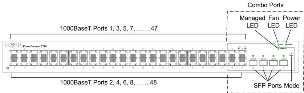
Figure 2-7. Panneau avant du PowerConnect 2748
