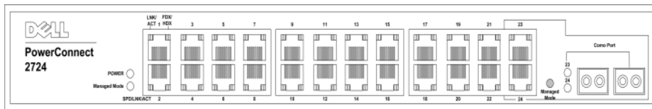
Figure 1-3. Panneau avant du PowerConnect 2724
